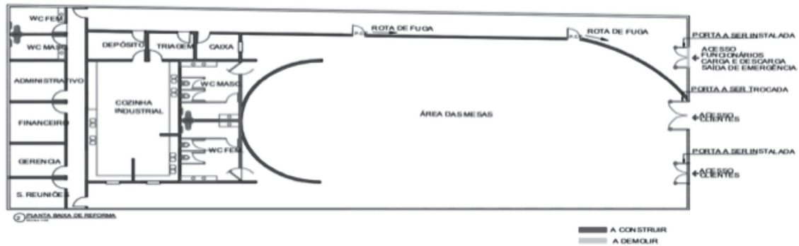
Imagem 5 – Planta baixa de reforma do trapiche
